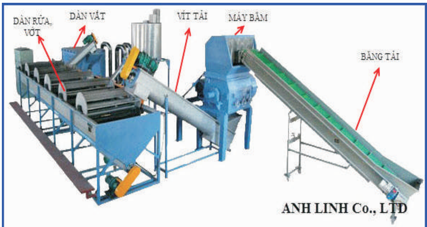
DÂY CHUYỀN BẮM RỬA NHỰA PHẾ LIỆU
