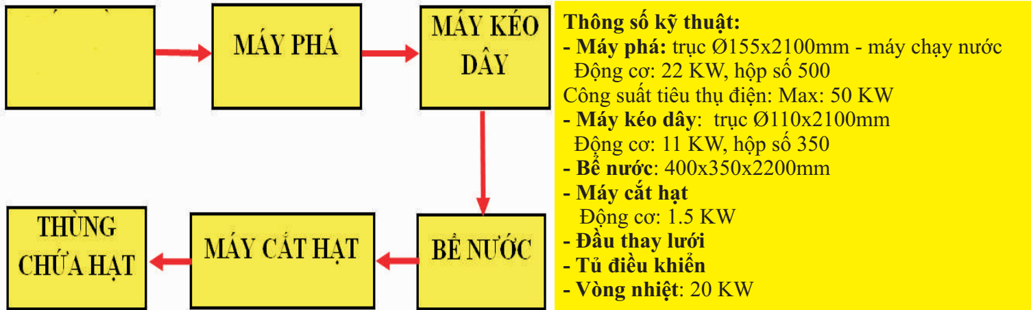
SƠ ĐỒ KHỐI DÂY CHUYỀN TẠO HẠT NHỰA TÁI SINH
